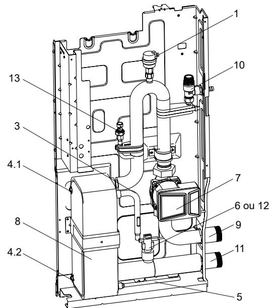
Une unité de 8 à 16 kW sans réchauffeur de secours
