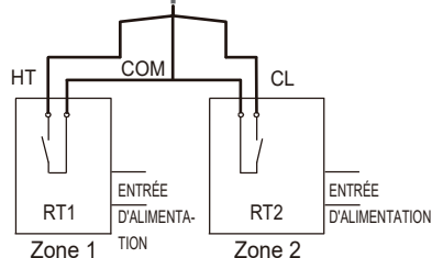
Méthode C (commande de zone double)
