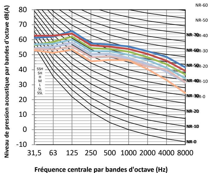
III. 8.15 : Niveaux par bandes d'octave MIH560T1N18 (KPDUF-560 DN5.0)
