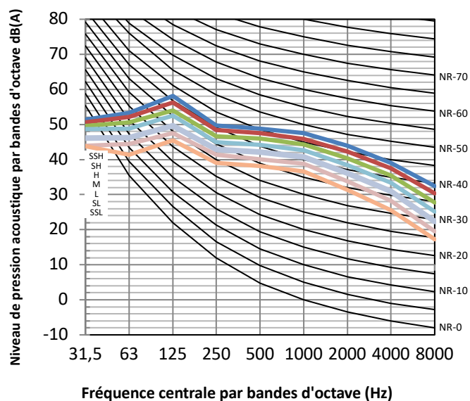
III. 8.12 : Niveaux par bandes d'octave MIH280T1N18
